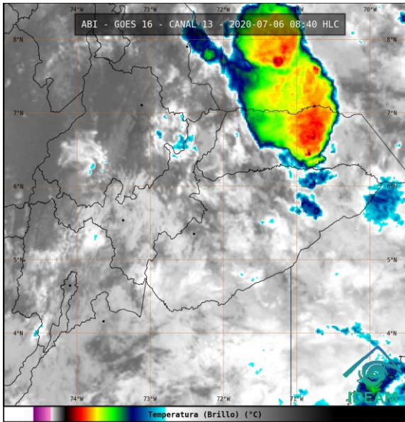
Imagen satelital infrarrojo GOES 16 Julio 06 de 2020 – Hora 8:40 HLC.
